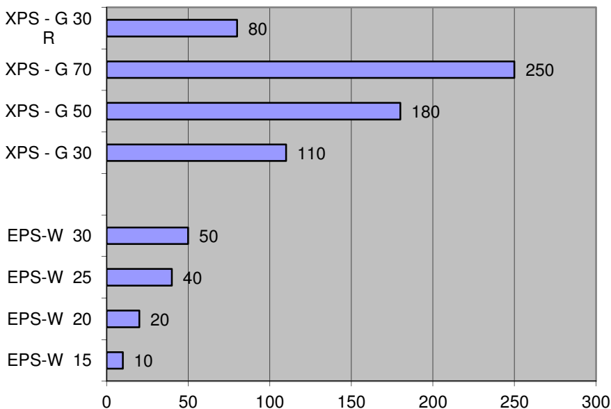
Druckspannungen bei 2 % Stauchung
